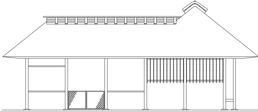
西立面図 S=1/50(1/100)
