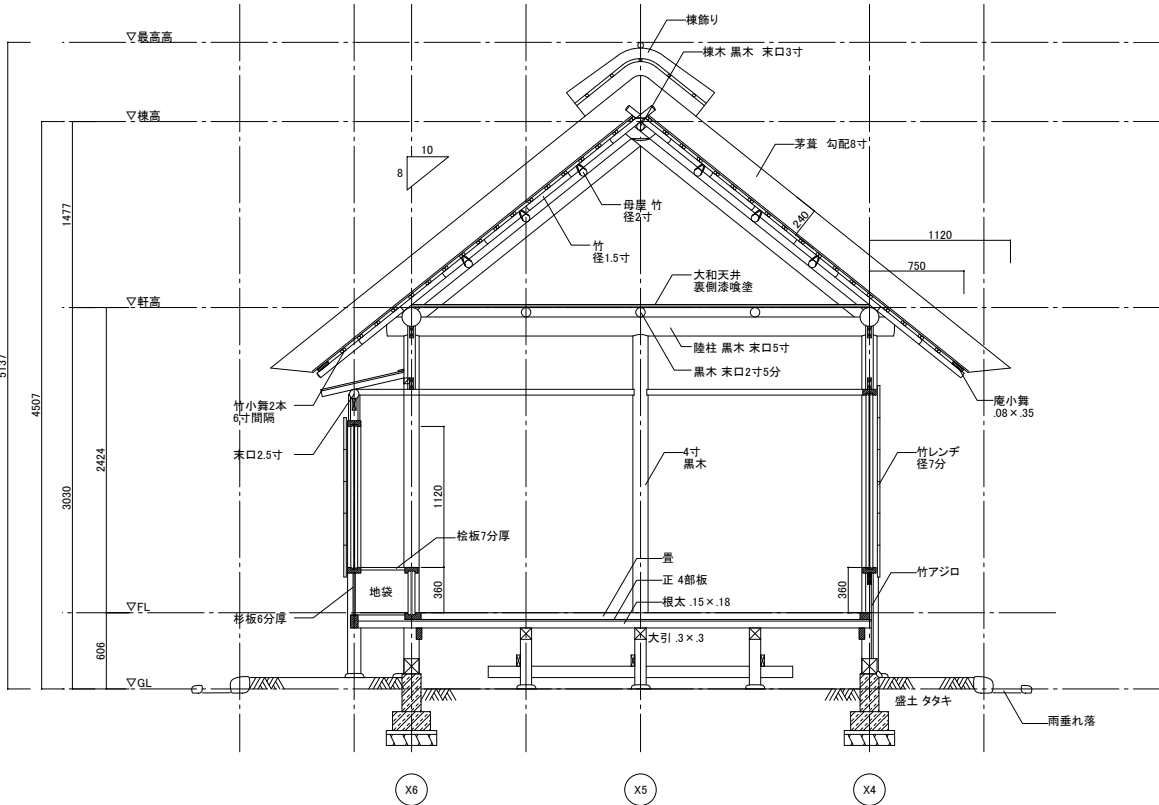
A 断面図 S=1/30(1/50)
