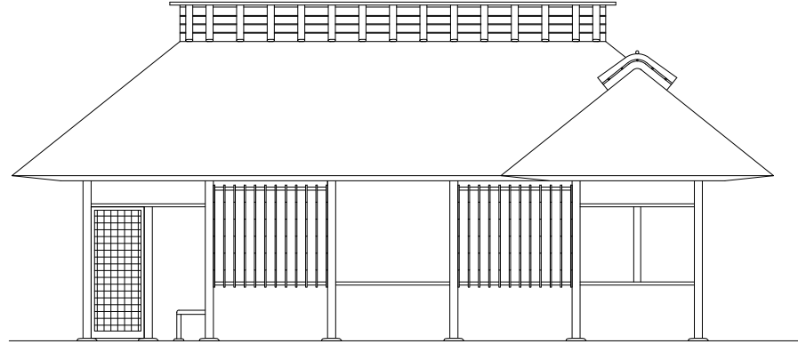
北立面図 S=1/50(1/100)
