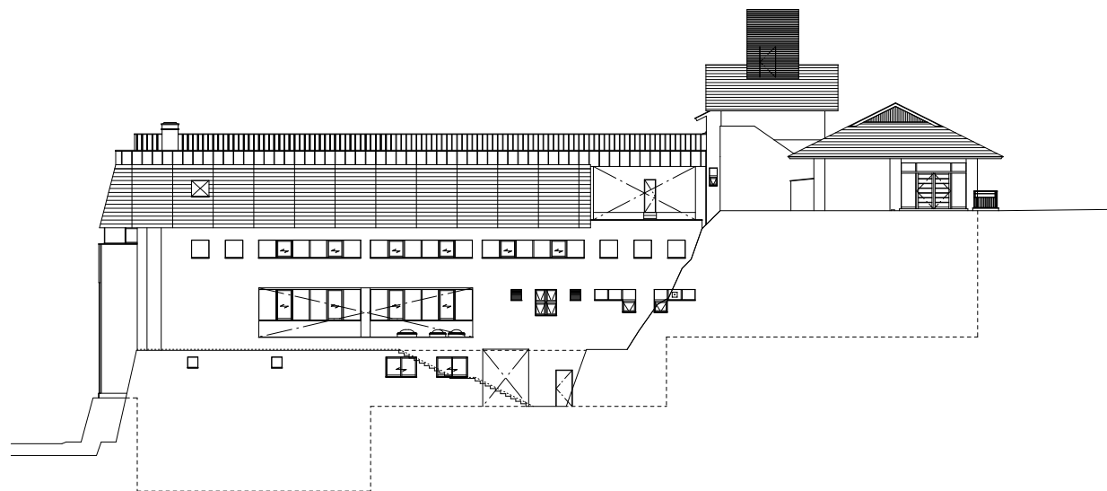
北立面図 S=1/200(1/400)
