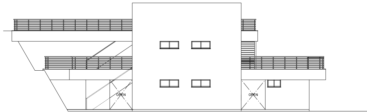
東立面図 S=1/100(1/200)
