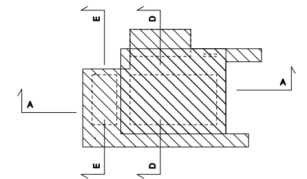
断面位置 配置図 S=1/200(1/400)
