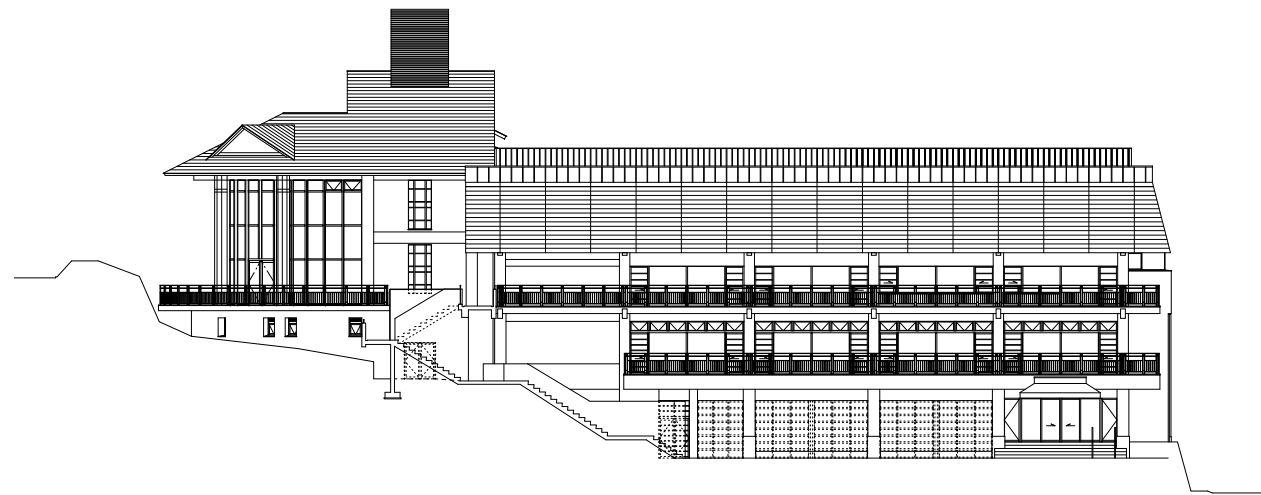
南立面図 S=1/200(1/400)
