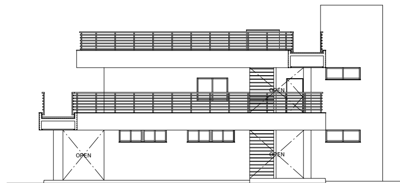
北立面図 S=1/100(1/200)
