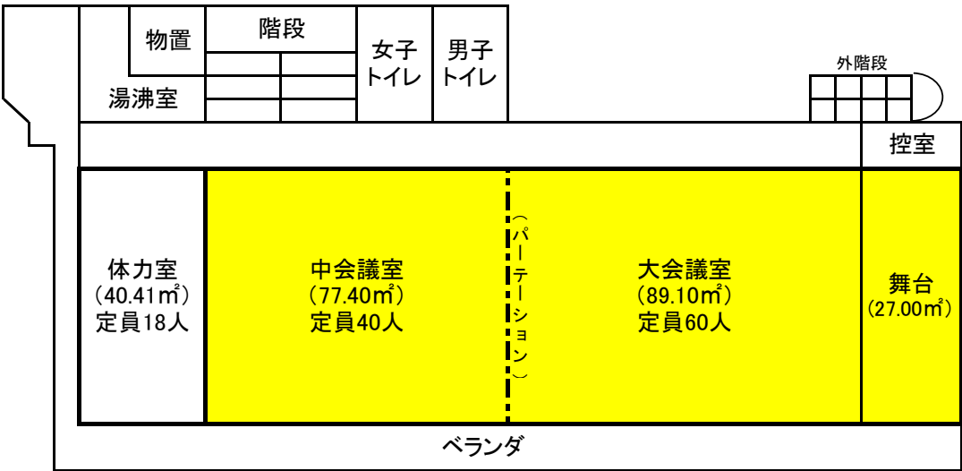
2階 平面図
