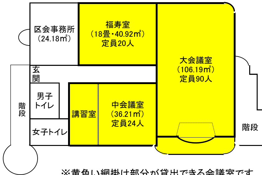
2階 平面図
