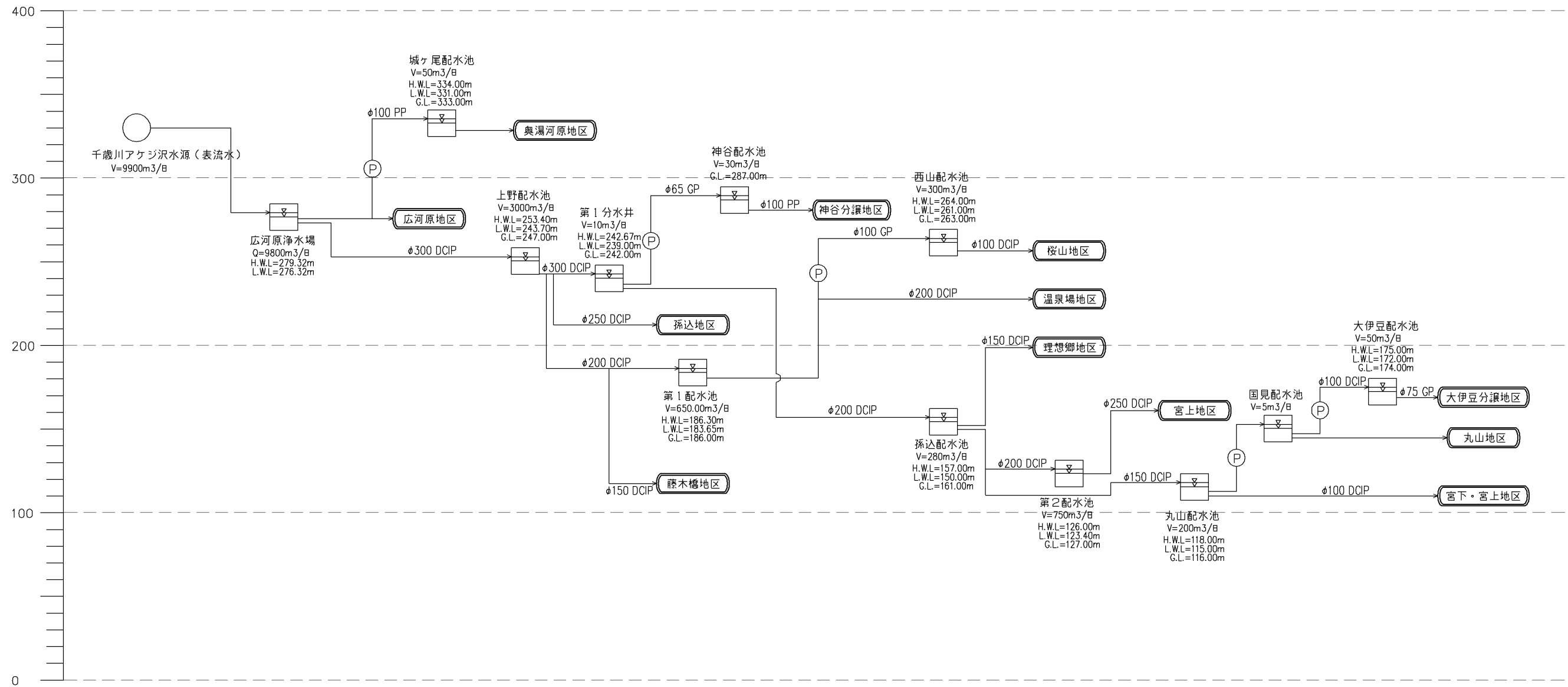
図 2.4 湯河原上水道施設水位高低図
